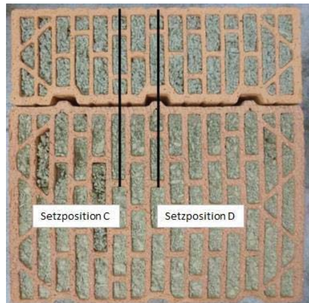
Bild 2: Setzpositionen der Dübel in wärmedämmenden PlanHLz
